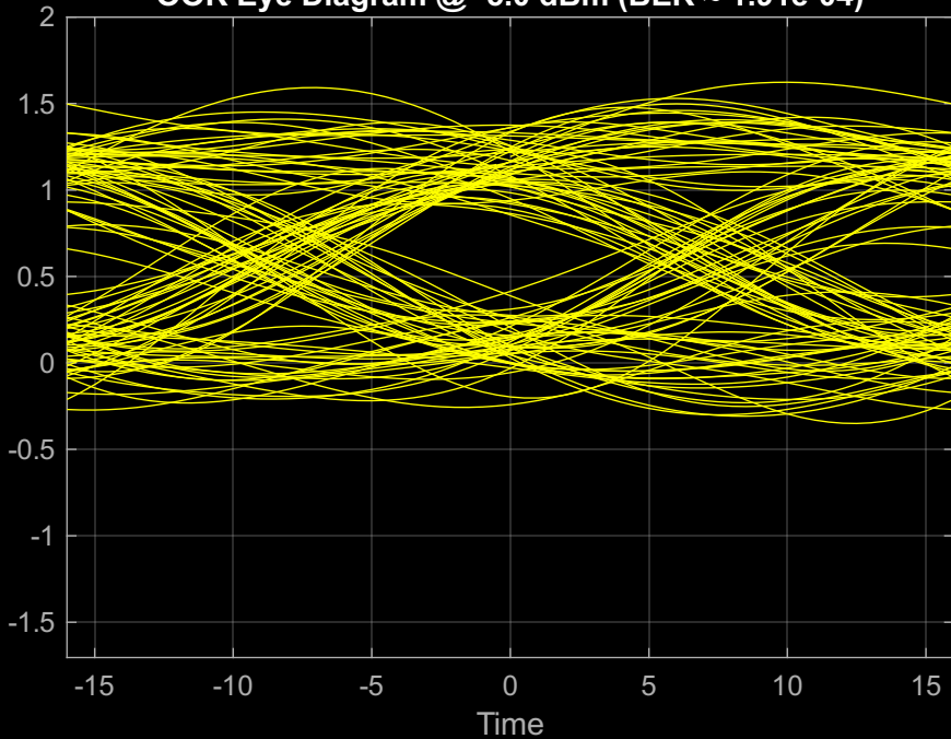
OOK Eye Diagram @ -5.0 dBm (BER \approx 1.91\text{e-}04 )
